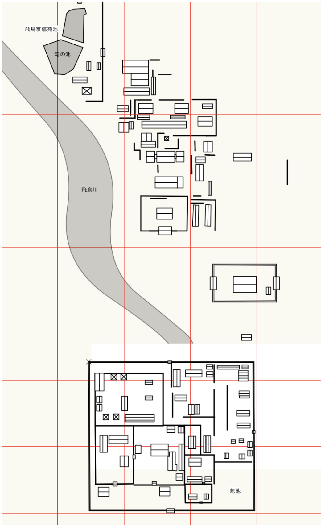
上図／嶋宮遺構復原図（私案） 下図／長屋王邸復原図（奈文研） 100mx100m
